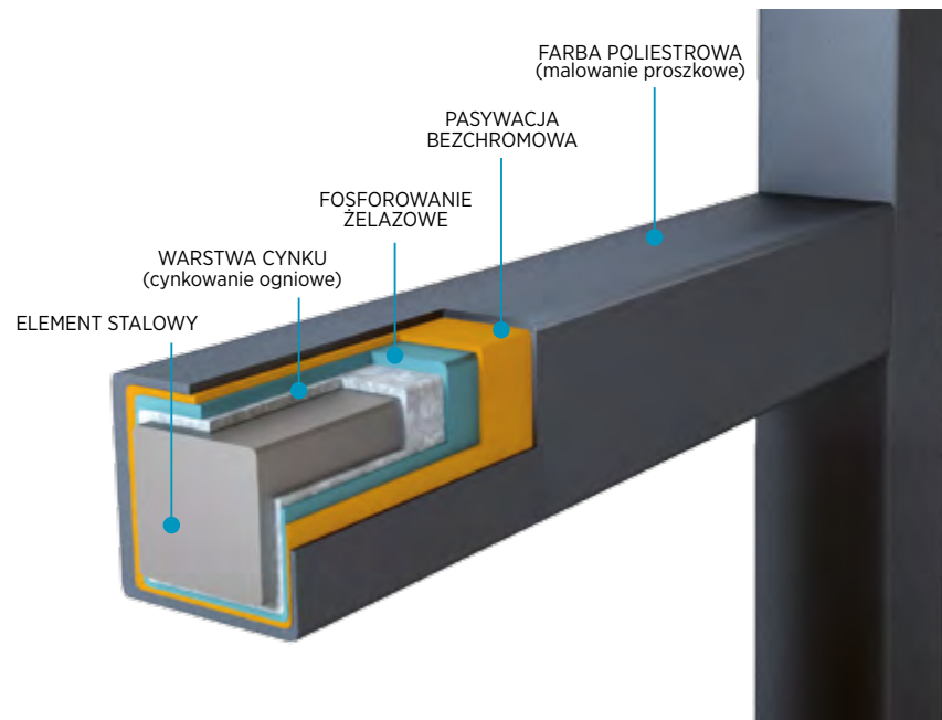
Przekrój przez element zabezpieczony w systemie DUPLEX
